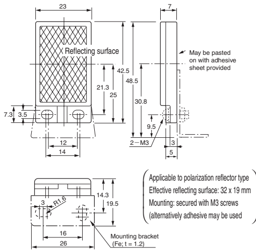
(K-71 reflector)
