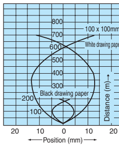
GSR05RSN · GSR05RN
